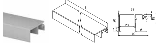
Für Bodenmontage-Profile
