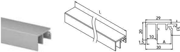
Für Bodenmontage-Profile
