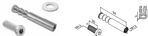
Ankerstange
